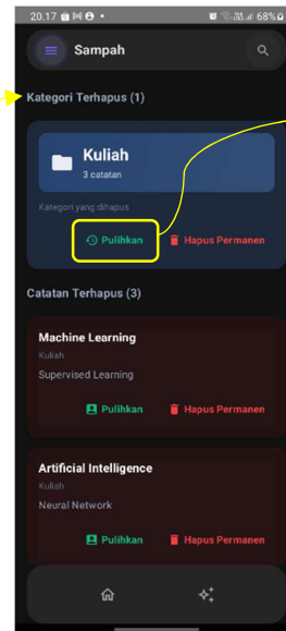
Gambar 20 Halaman Sampah
